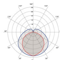
Distribuzione fotometrica
